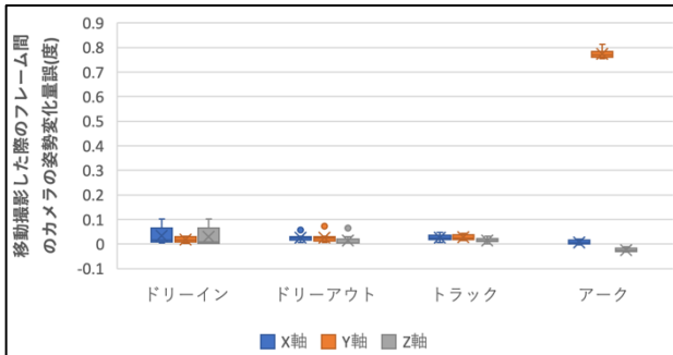
図7 フレーム間のカメラの姿勢変化量の誤差の平均
