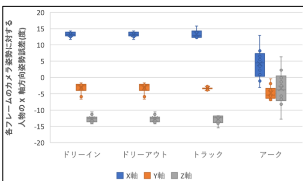
図9 カメラ姿勢に対する人物の X 軸方向姿勢誤差の平均
