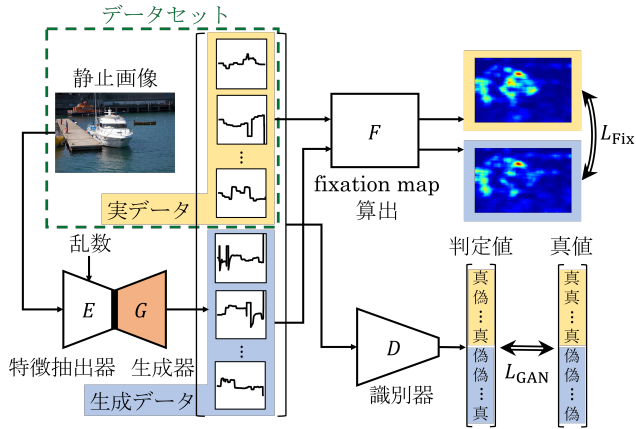
図 1: 眼球運動を生成する GAN
