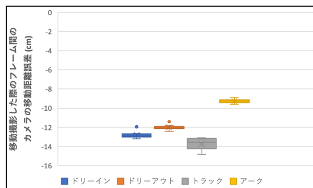
図5 フレーム間のカメラの移動距離誤差の平均
