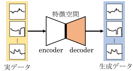
図 2: 眼球運動を生成する autoencoder
