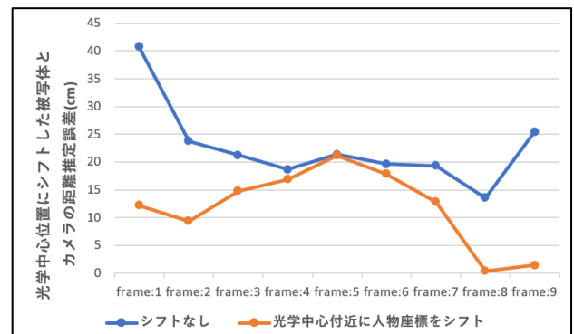
図11 被写体位置におけるカメラと被写体の距離推定誤差
