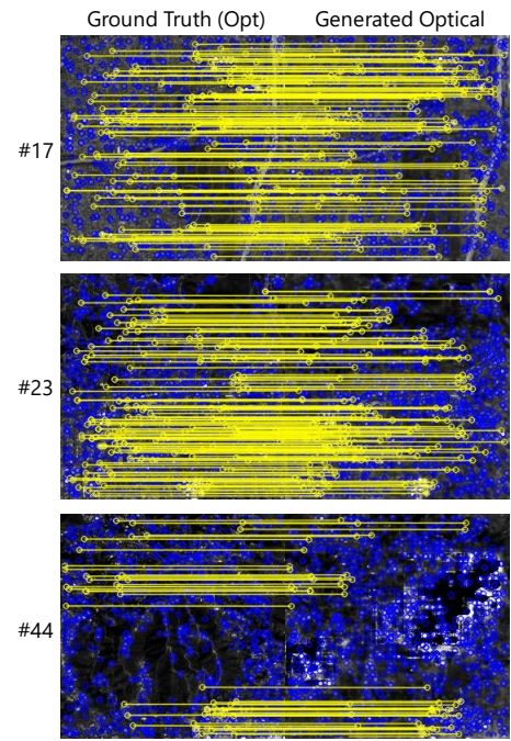
図 6 対応点探索の結果. PSNR 最悪値のケースにおいて, 崩壊した領域では局所的な特徴の対応は検出されないが, 残りの箇所に多くの対応点が発見されている.
